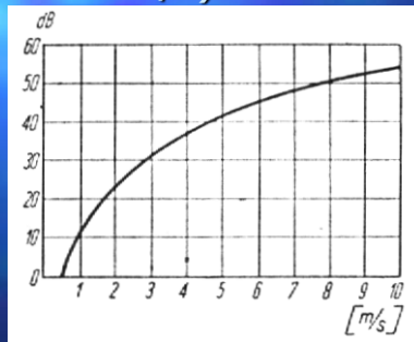
Zależność intensywności szumu od prędkości przepływu powietrza
